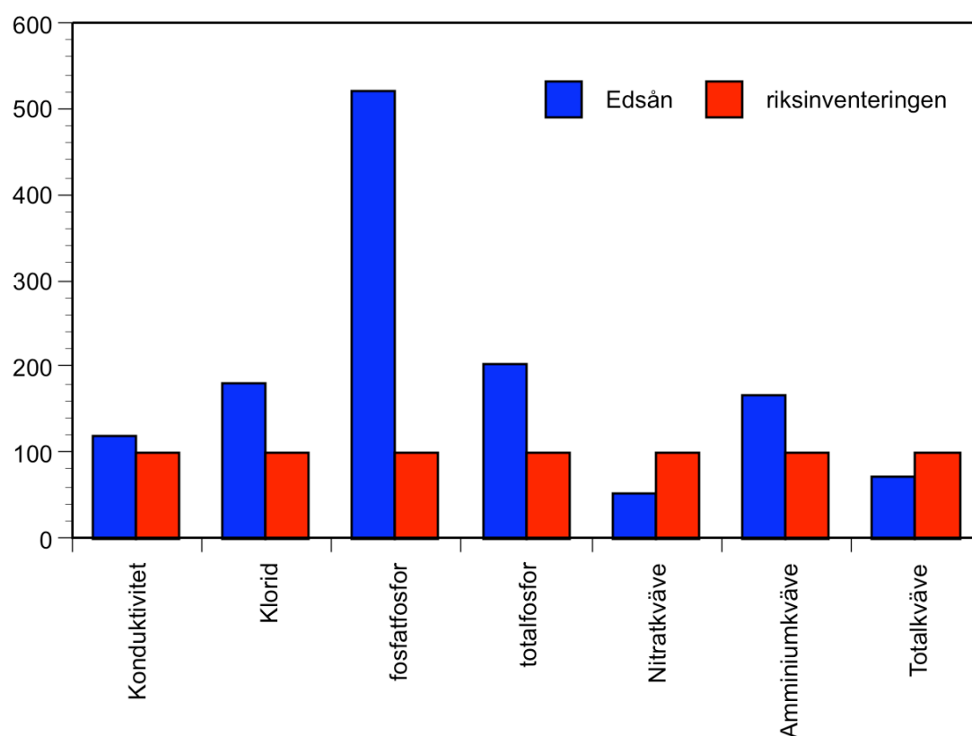
Figur 14. En jämförelse mellan mätvärden (oktober-november) från riksinventeringen (SLU, 2000) och Edsån.
