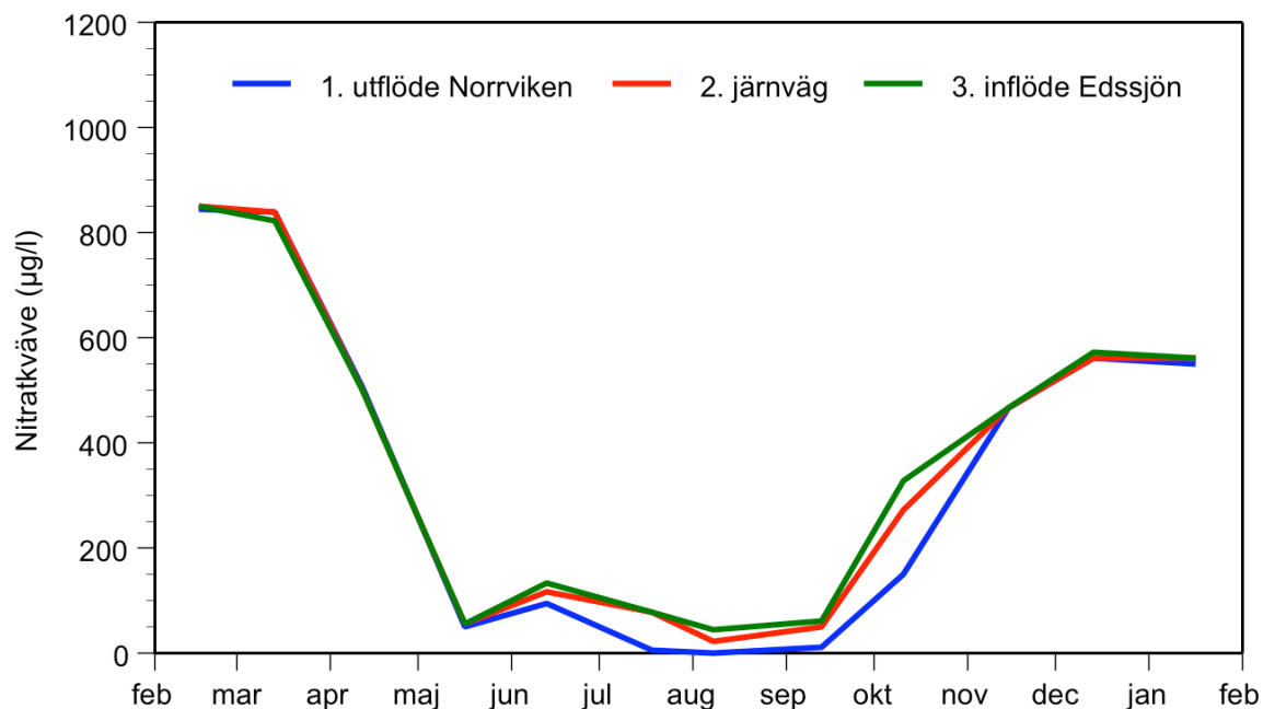
Figur 12. Nitratkvävehalten vid de tre provpunkterna i Edsån under perioden februari 2005- januari 2006.
