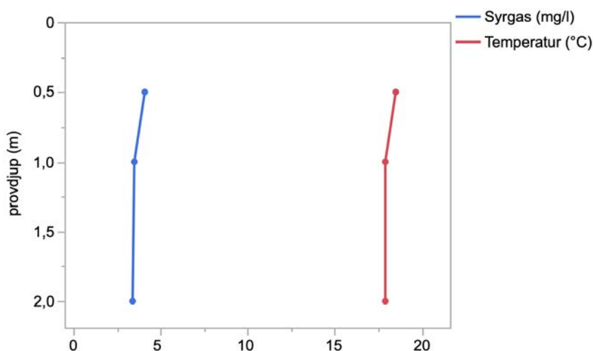
Figur 9. Temperatur- och syrgasprofil i Gullsjön den 29 augusti 2018
